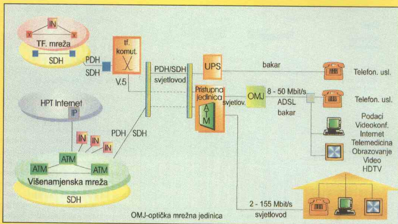
Slika 8. Ciljna struktura pristupne mreže u Hrvatskoj
